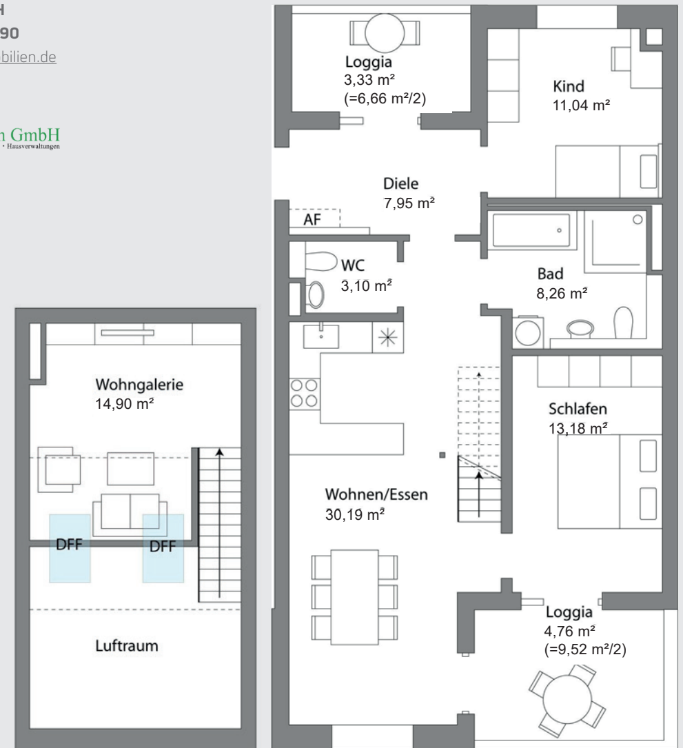
2. Obergeschoss
